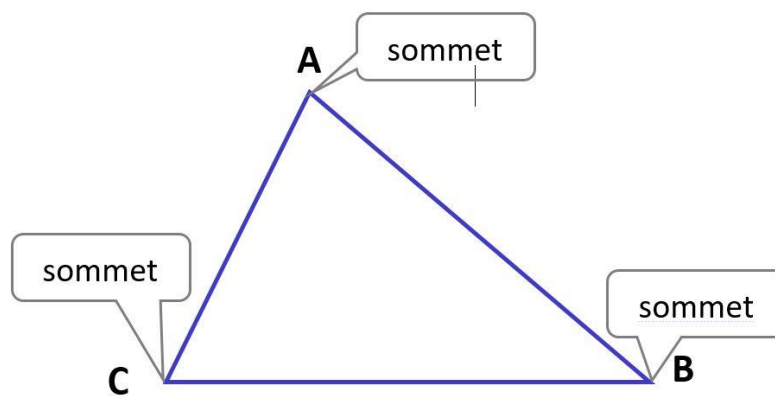
Les 3 sommets d'un triangle : A, B et C
