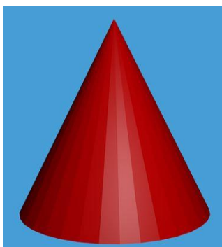
Cône (image Pixabay)
