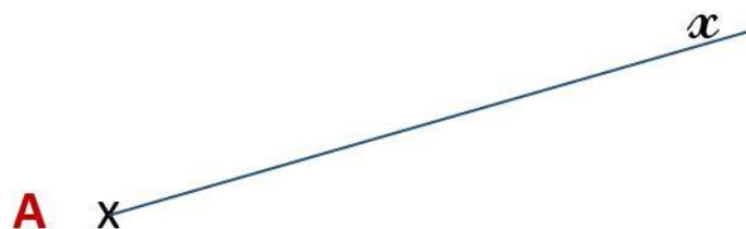
La demi-droite Ax
