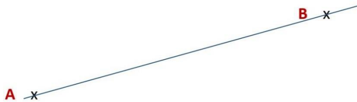
La droite (AB)
