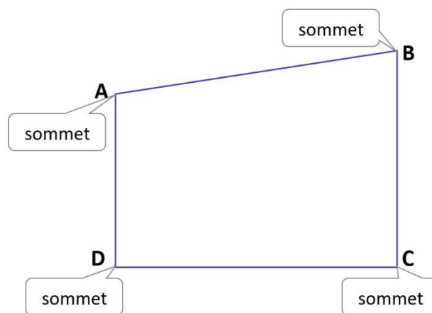
Les 4 sommets d'un quadrilatère : A, B, C et D
