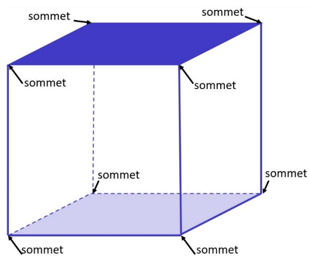
Les 8 sommets d'un cube
